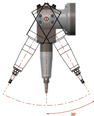
VERTICAL SET UP B AXIS SENKRECHTE KONFIGURATION
